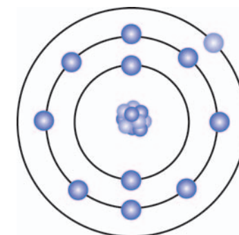
SODIUM ATOM
